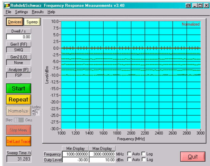
Fig. 2 Main Menu
